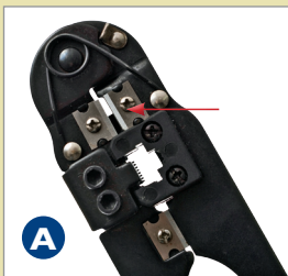
Identificando as lâminas de decapagem do cabo.
