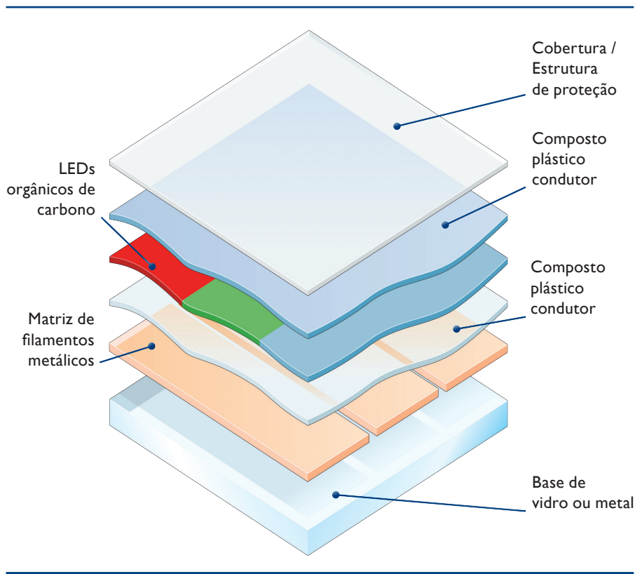
Figura 96 Camadas do monitor OLED.
