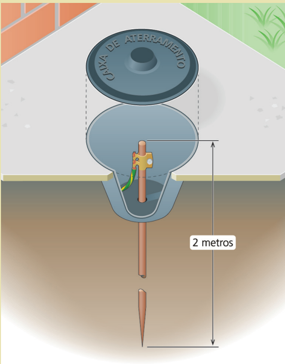
Figura 7 Aterramento com barra de cobre.
