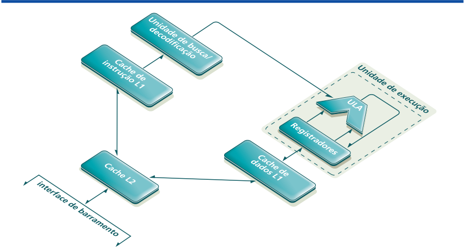
Figura 4 Componentes de um processador.
